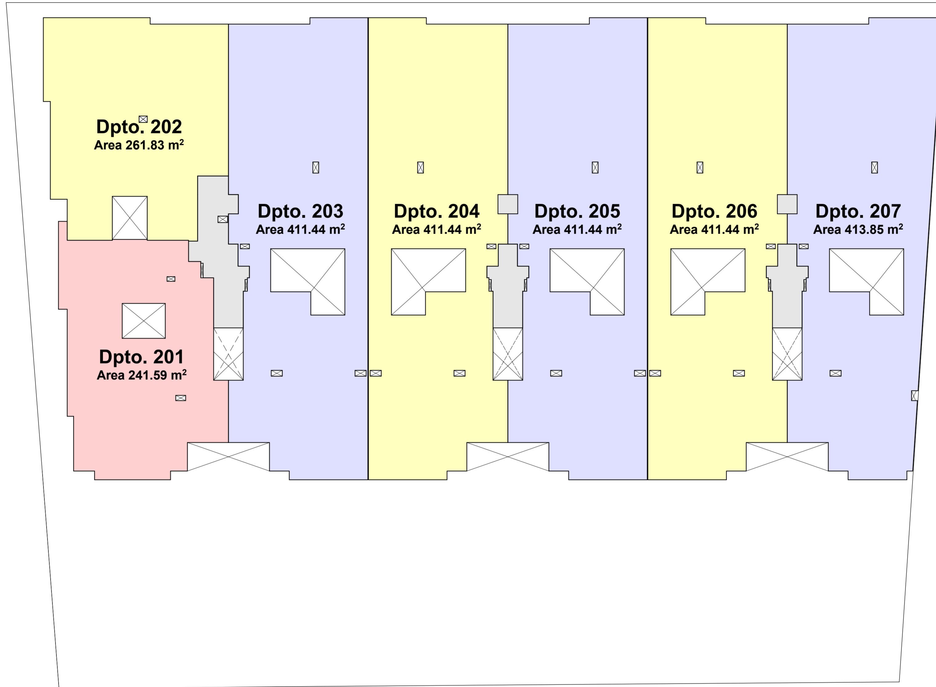
PLANTA SEGUNDO PISO
